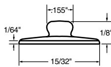
106-W04-1T STUD
