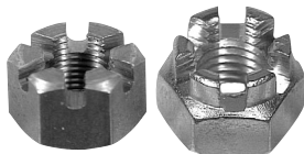
DIN 935 Slotted and Castellated Hexagon Nuts Écrous hexagonaux à créneaux pg. C17 ~ISO 7035/7036/7037
