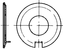
DIN 432 External Tab Washers Plaques d'arrêt avec ergot pg. D13
